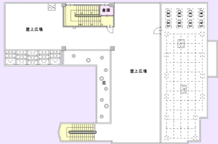
4階平面図
